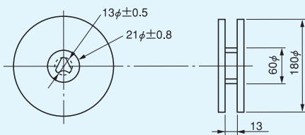
リール寸法図
