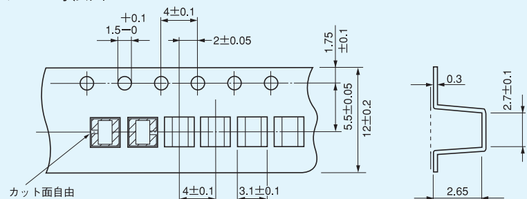
テープ寸法図
