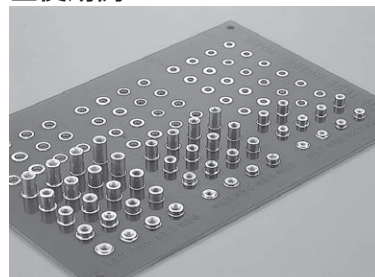
リフロー後、吸着用フィルムをはずした状態
