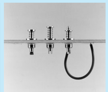
プリント基板に取付けた場合
