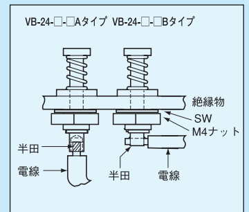
樹脂に取付けた場合
