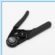
圧着工具本体 ■品番 OMXT-1
