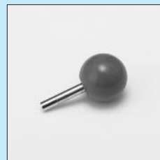
ハウジングにソケット、ピンを圧入する工具 ■品番 PCX-1 (先端チップP-3)
